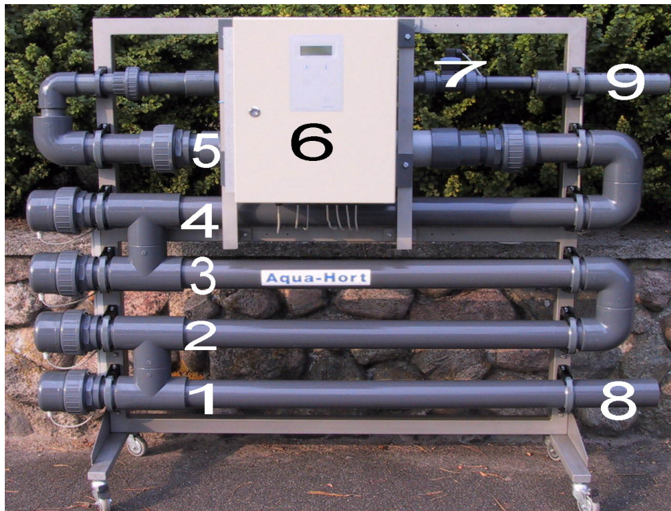
Uitleg (Standard Buis Unit): 1) Electrode 1, 2) Electrode 2, 3) Electrode 3, 4) Electrode 4, 5) Electromagneet, 6) Control Box, 7) Flow meter, 8) Water in, 9) Water uit.
